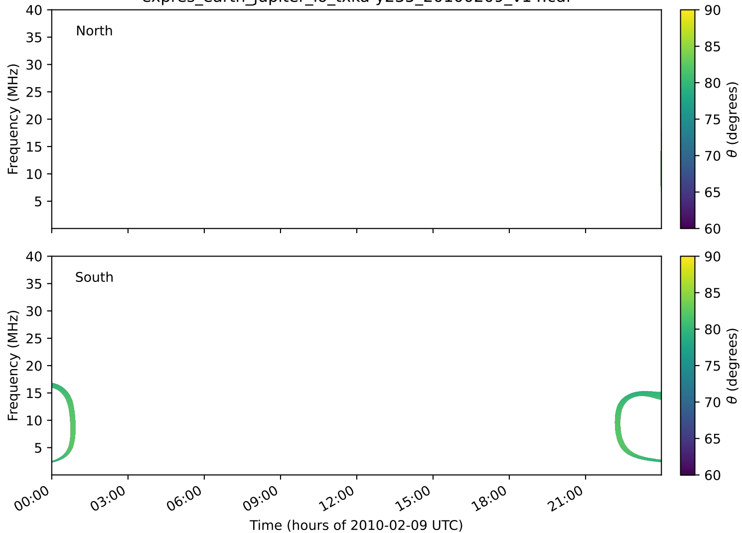
expres_earth_jupiter_io_txka-y235_20100209_v14.cdf
