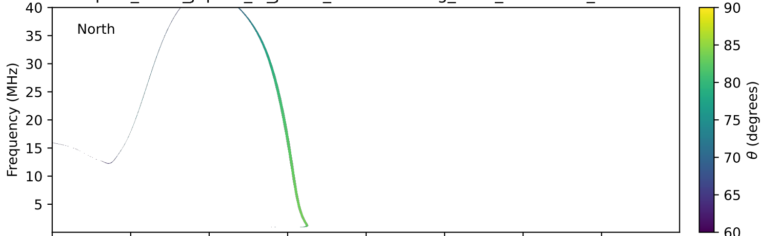
expres_earth_jupiter_io_jrm09_lossc-wid1deg_3kev_19930209_v11.cdf
