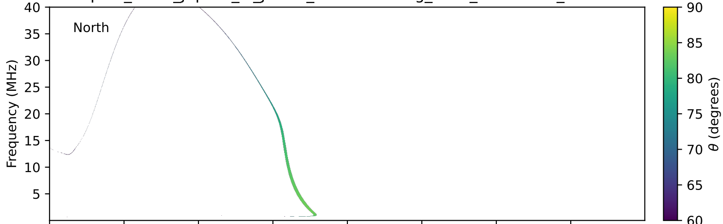
expres_earth_jupiter_io_jrm09_lossc-wid1deg_3kev_19921209_v11.cdf
