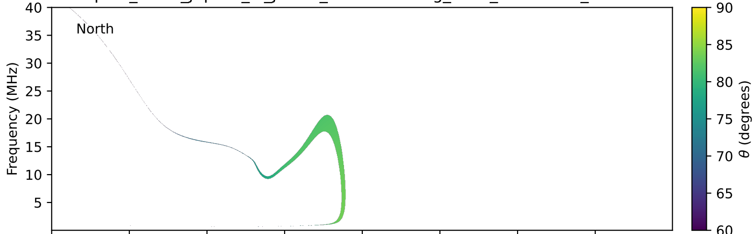
expres_earth_jupiter_io_jrm09_lossc-wid1deg_3kev_19910209_v11.cdf
