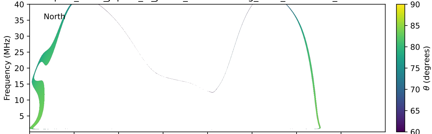
expres_earth_jupiter_io_jrm09_lossc-wid1deg_3kev_19900209_v11.cdf
