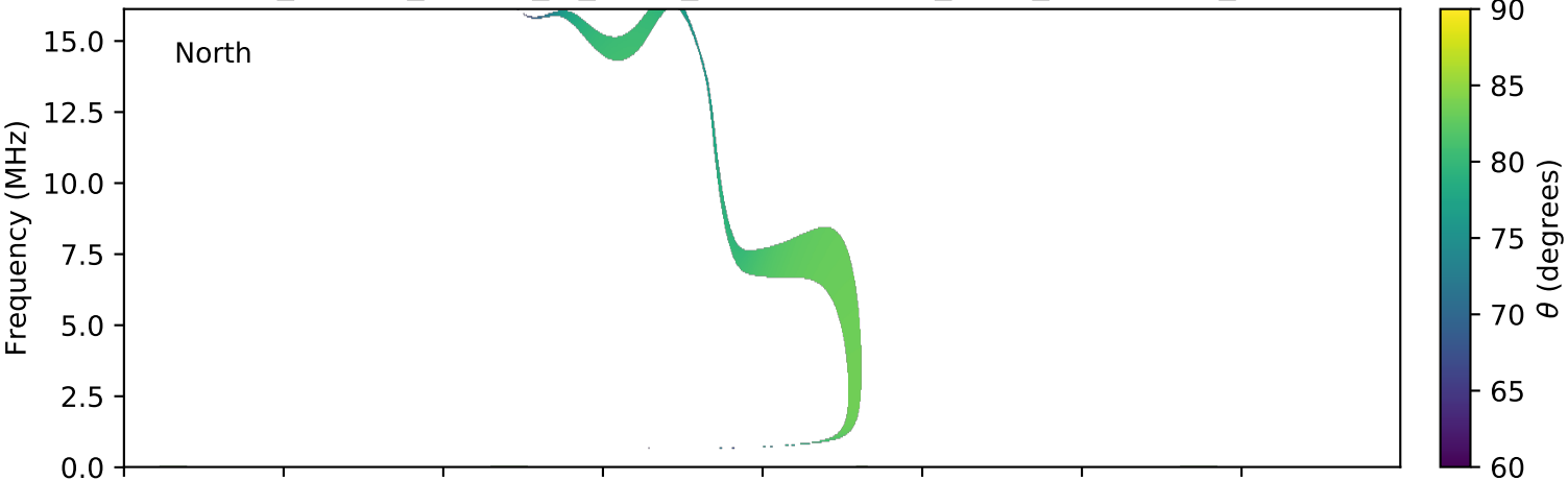
expres_cassini_jupiter_io_isaac_lossc-wid1deg_3kev_20020620_v01.cdf
