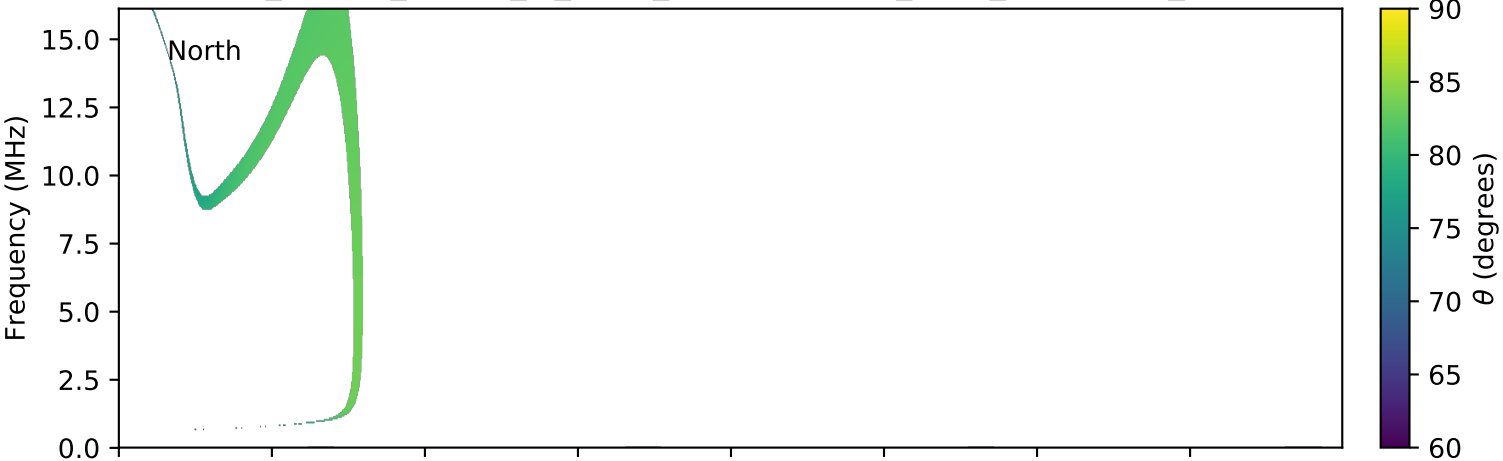
expres_cassini_jupiter_io_isaac_lossc-wid1deg_3kev_20020608_v01.cdf
