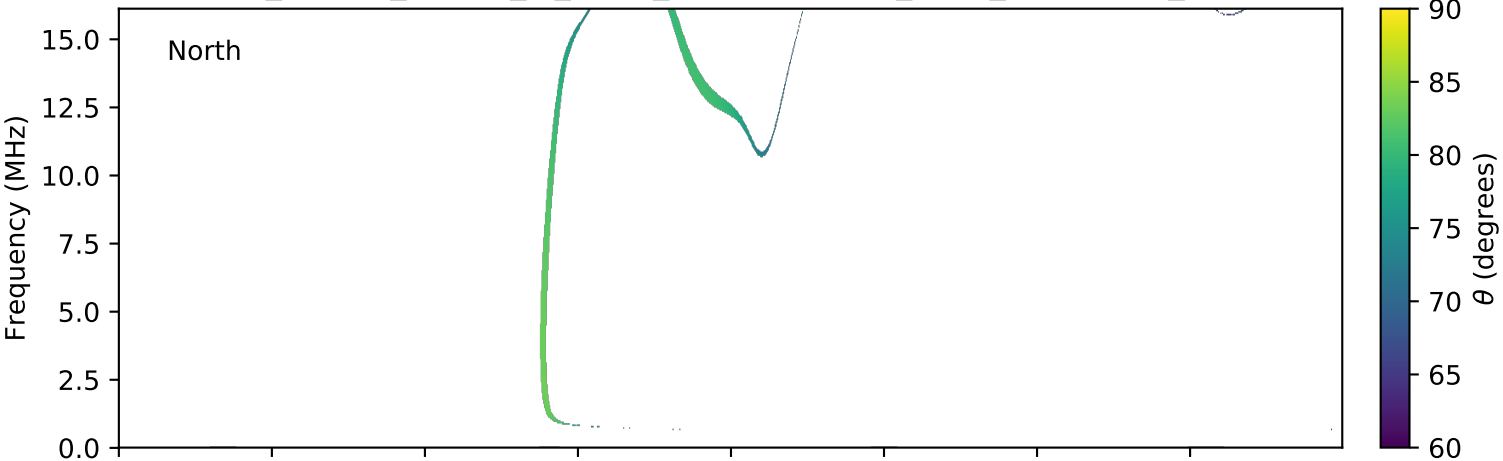
expres_cassini_jupiter_io_isaac_lossc-wid1deg_3kev_20020607_v01.cdf
