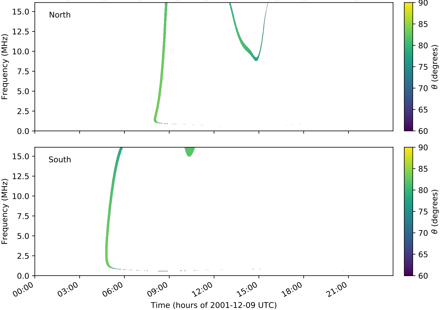
expres_cassini_jupiter_europa_isaac_lossc-wid1deg_3kev_20011209_v01.cdf
