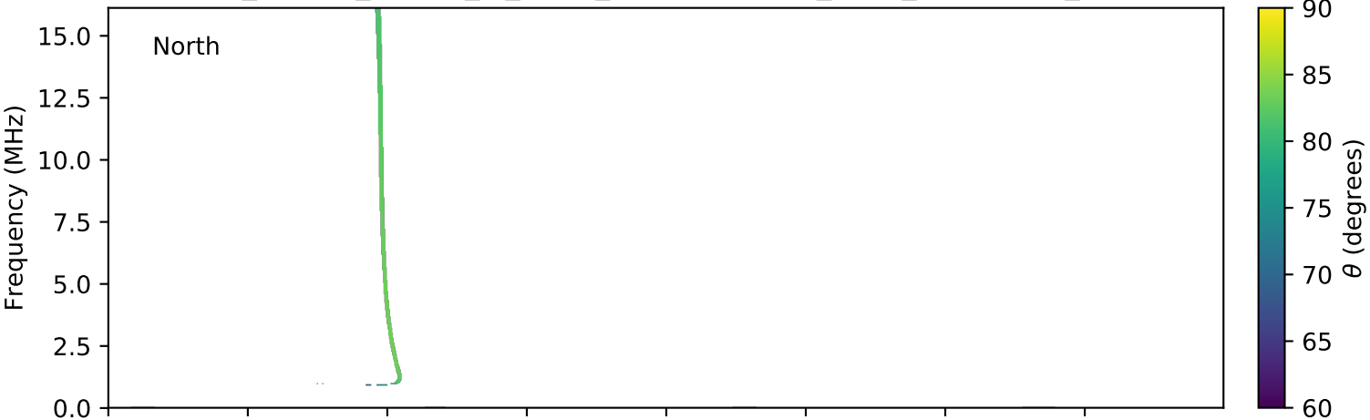
expres_cassini_jupiter_io_isaac_lossc-wid1deg_3kev_20010411_v01.cdf
