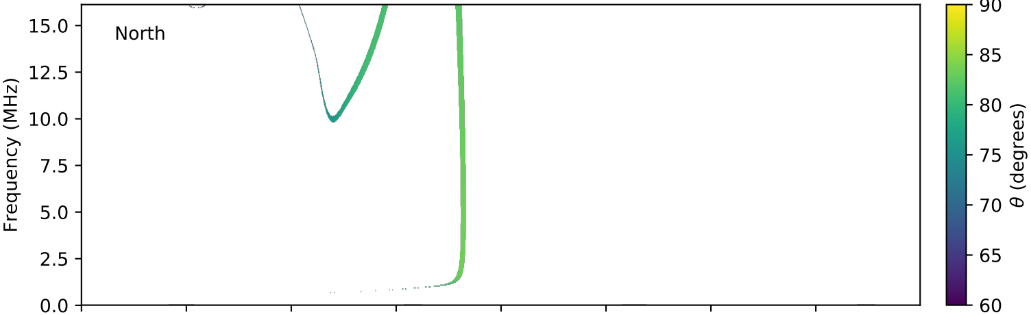
expres_cassini_jupiter_io_isaac_lossc-wid1deg_3kev_20010402_v01.cdf
