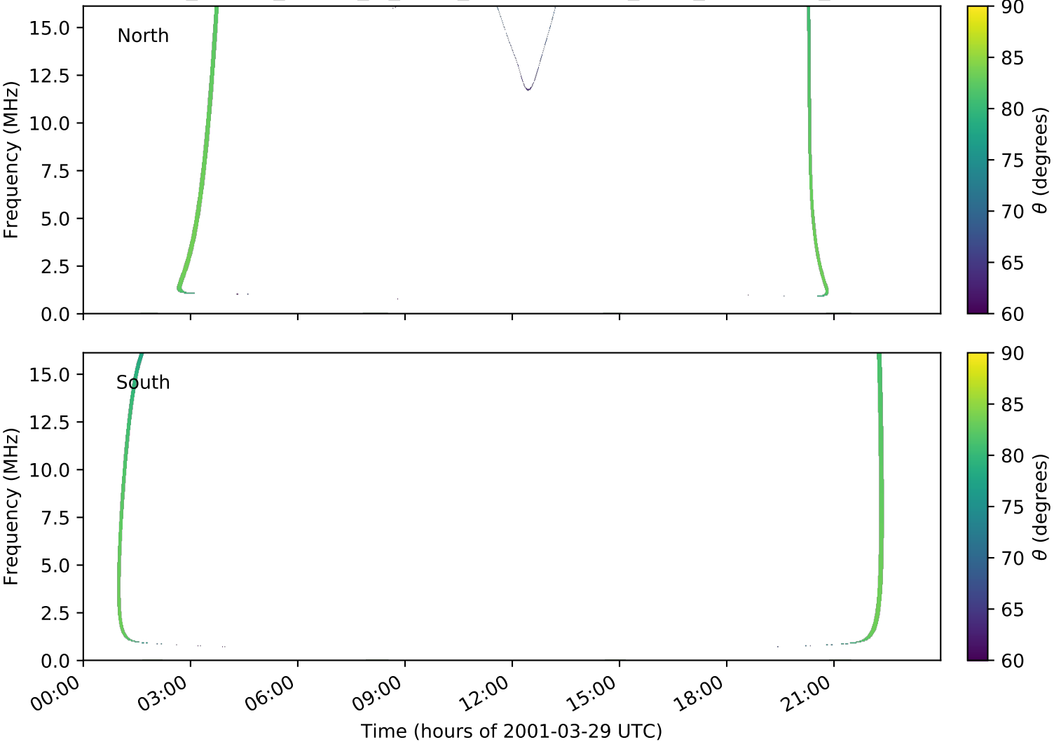
expres_cassini_jupiter_io_isaac_lossc-wid1deg_3kev_20010329_v01.cdf
