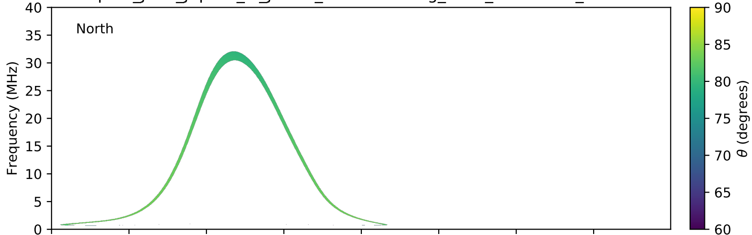
expres_juno_jupiter_io_jrm09_lossc-wid1deg_3kev_20211217_v11.cdf
