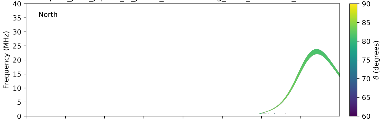
expres_juno_jupiter_io_jrm09_lossc-wid1deg_3kev_20211211_v11.cdf
