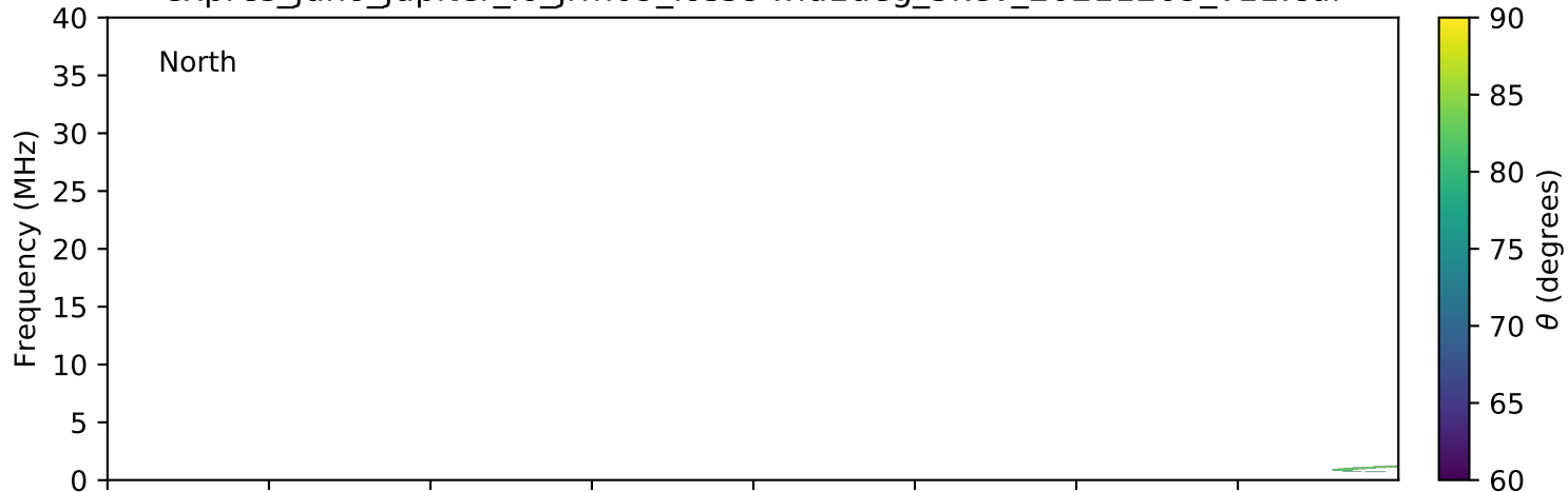
expres_juno_jupiter_io_jrm09_lossc-wid1deg_3kev_20211209_v11.cdf
