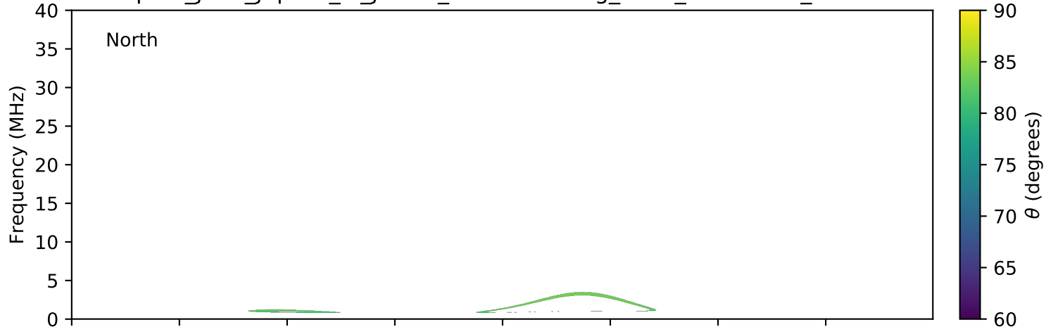
expres_juno_jupiter_io_jrm09_lossc-wid1deg_3kev_20211201_v11.cdf
