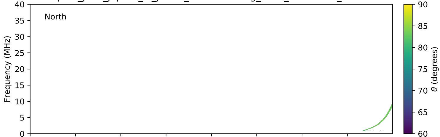
expres_juno_jupiter_io_jrm09_lossc-wid1deg_3kev_20211116_v11.cdf
