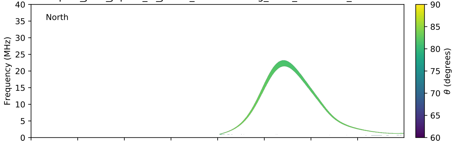
expres_juno_jupiter_io_jrm09_lossc-wid1deg_3kev_20211028_v11.cdf
