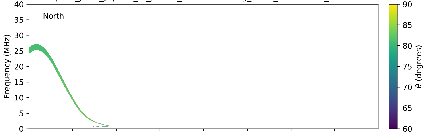
expres_juno_jupiter_io_jrm09_lossc-wid1deg_3kev_20211027_v11.cdf
