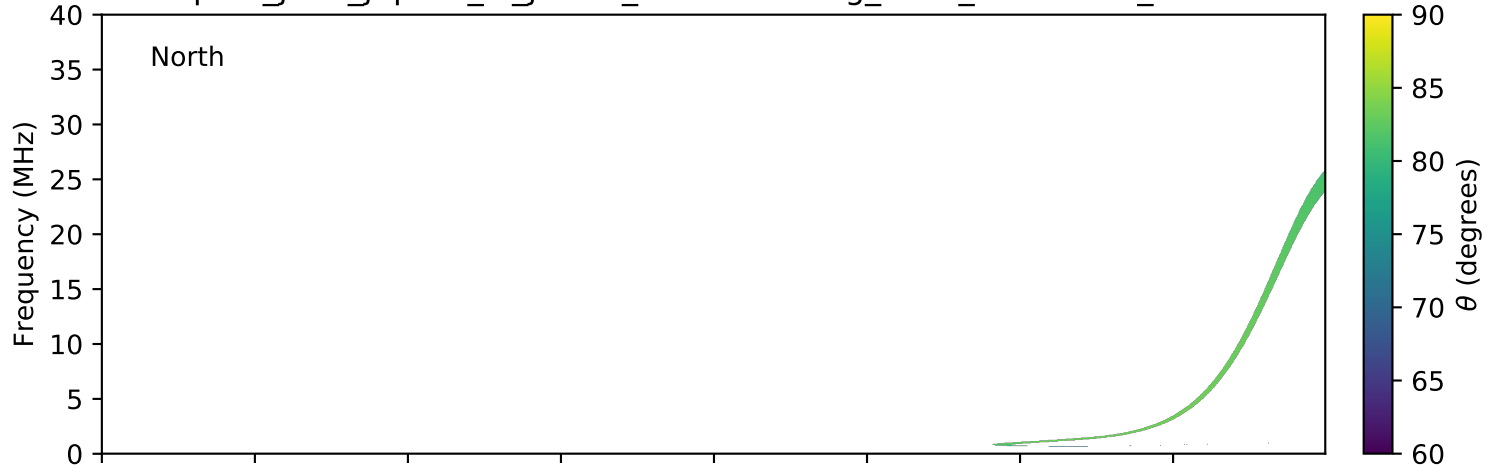
expres_juno_jupiter_io_jrm09_lossc-wid1deg_3kev_20211026_v11.cdf
