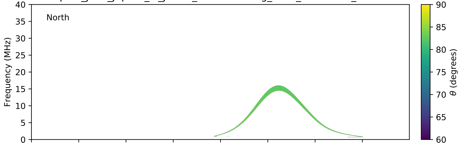
expres_juno_jupiter_io_jrm09_lossc-wid1deg_3kev_20211021_v11.cdf
