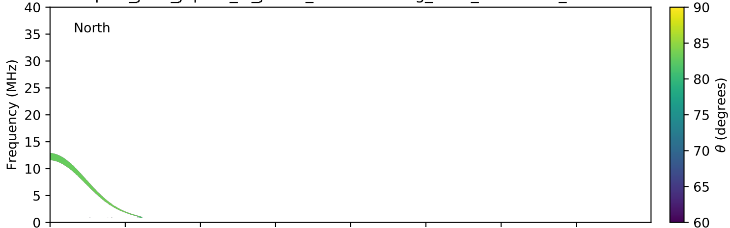
expres_juno_jupiter_io_jrm09_lossc-wid1deg_3kev_20211020_v11.cdf
