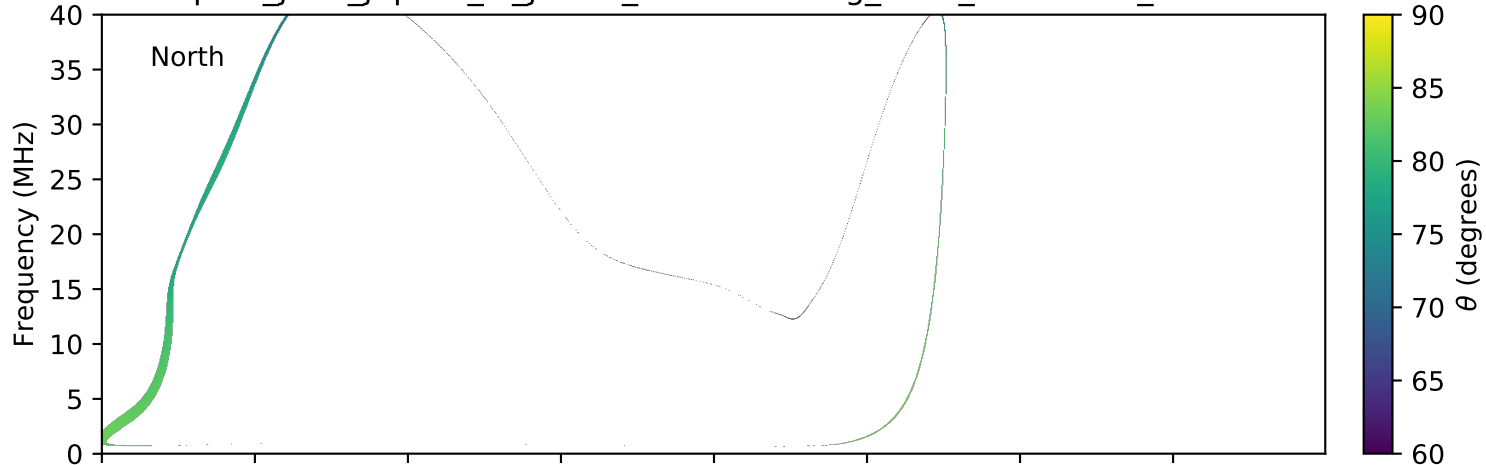
expres_juno_jupiter_io_jrm09_lossc-wid1deg_3kev_20211016_v11.cdf
