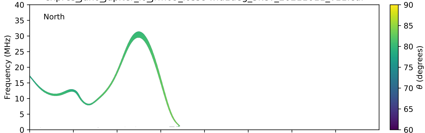
expres_juno_jupiter_io_jrm09_lossc-wid1deg_3kev_20211011_v11.cdf
