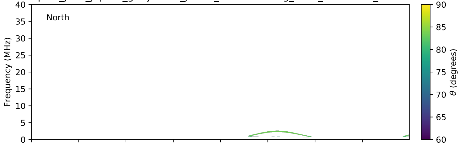
expres_juno_jupiter_ganymede_jrm09_lossc-wid1deg_3kev_20211021_v11.cdf
