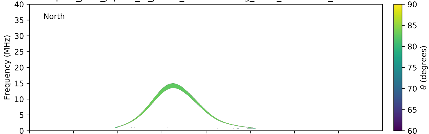
expres_juno_jupiter_io_jrm09_lossc-wid1deg_3kev_20210907_v11.cdf
