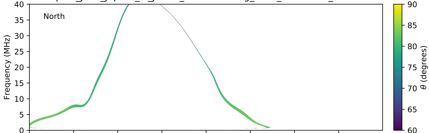
expres_juno_jupiter_io_jrm09_lossc-wid1deg_3kev_20210831_v11.cdf
