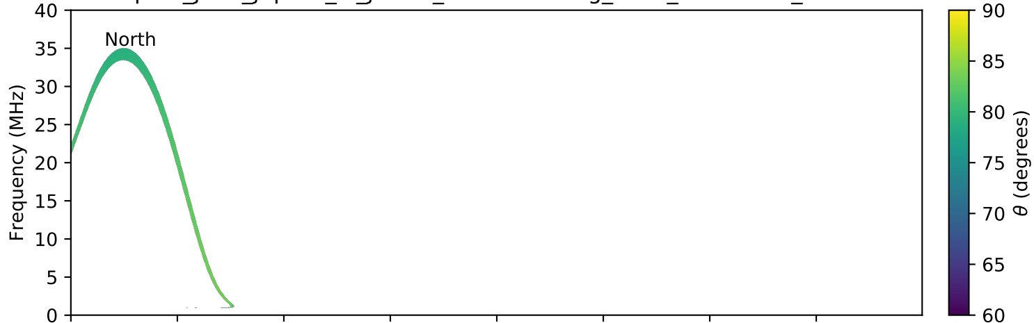
expres_juno_jupiter_io_jrm09_lossc-wid1deg_3kev_20210828_v11.cdf
