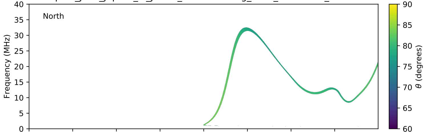
expres_juno_jupiter_io_jrm09_lossc-wid1deg_3kev_20210827_v11.cdf
