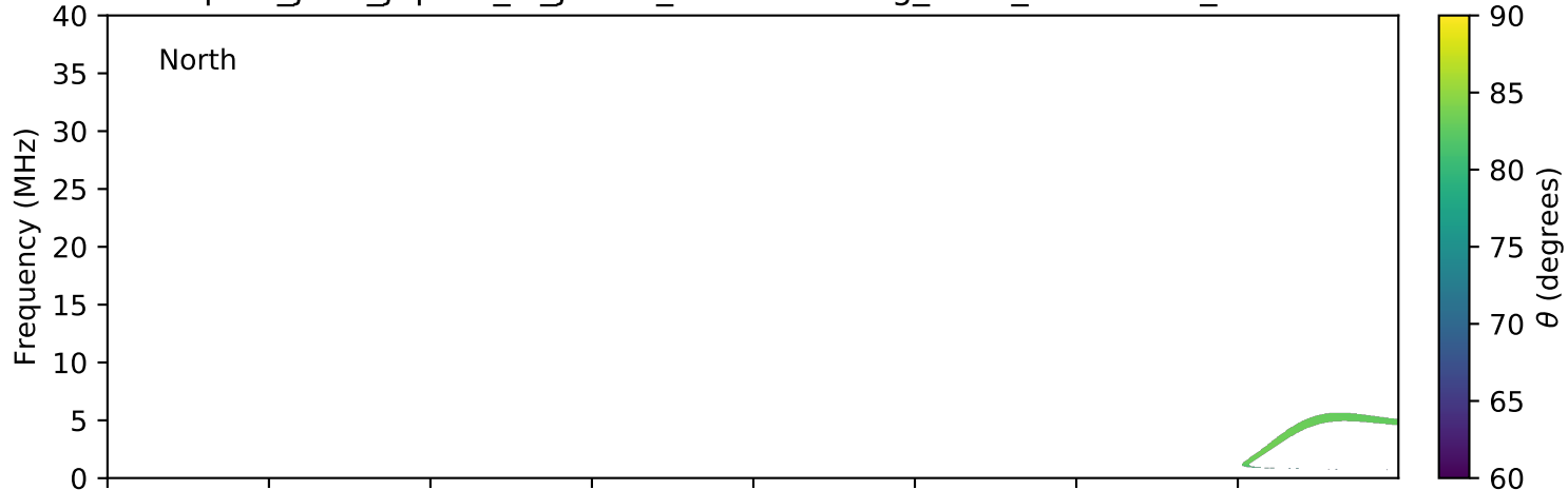
expres_juno_jupiter_io_jrm09_lossc-wid1deg_3kev_20210816_v11.cdf
