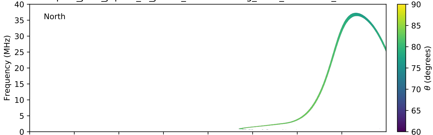
expres_juno_jupiter_io_jrm09_lossc-wid1deg_3kev_20210811_v11.cdf
