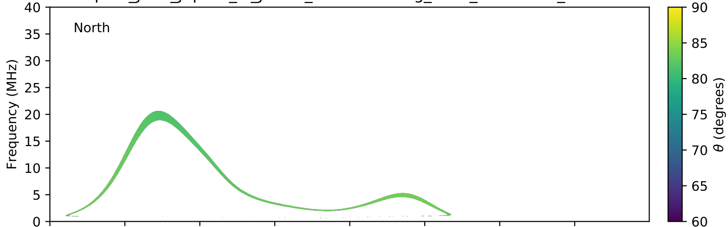
expres_juno_jupiter_io_jrm09_lossc-wid1deg_3kev_20210801_v11.cdf
