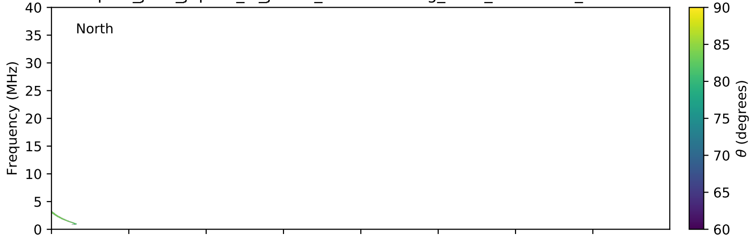
expres_juno_jupiter_io_jrm09_lossc-wid1deg_3kev_20210729_v11.cdf
