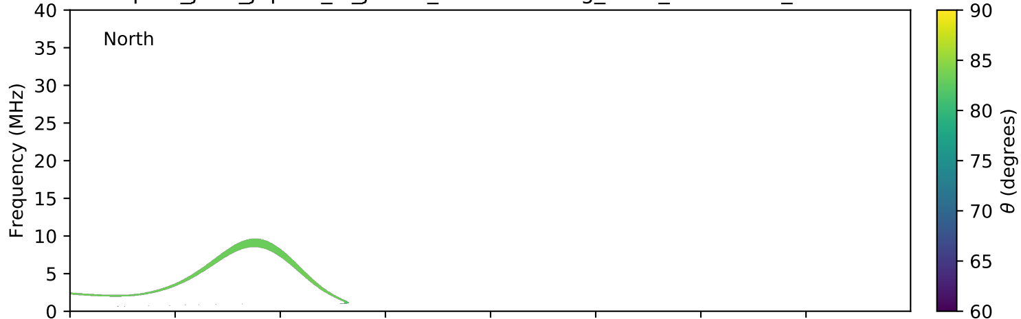
expres_juno_jupiter_io_jrm09_lossc-wid1deg_3kev_20210727_v11.cdf
