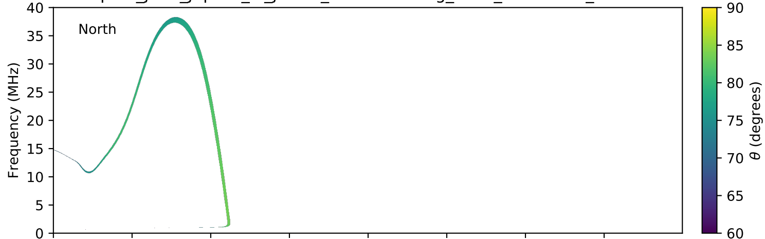
expres_juno_jupiter_io_jrm09_lossc-wid1deg_3kev_20210720_v11.cdf
