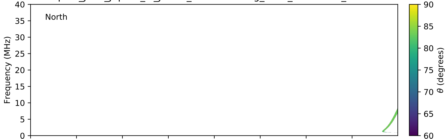
expres_juno_jupiter_io_jrm09_lossc-wid1deg_3kev_20210708_v11.cdf
