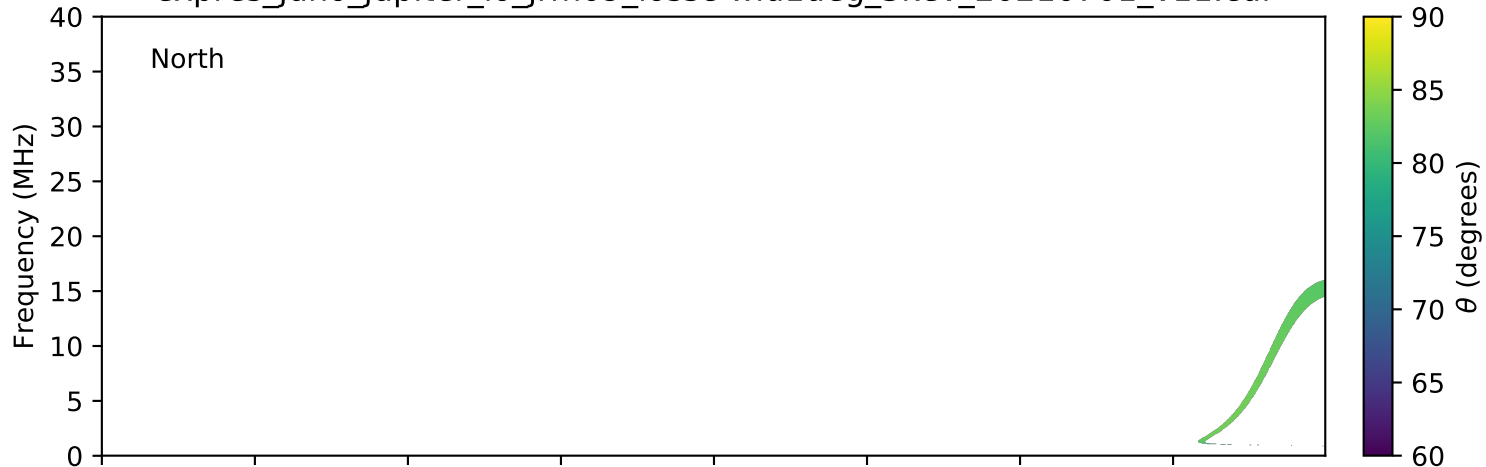
expres_juno_jupiter_io_jrm09_lossc-wid1deg_3kev_20210701_v11.cdf
