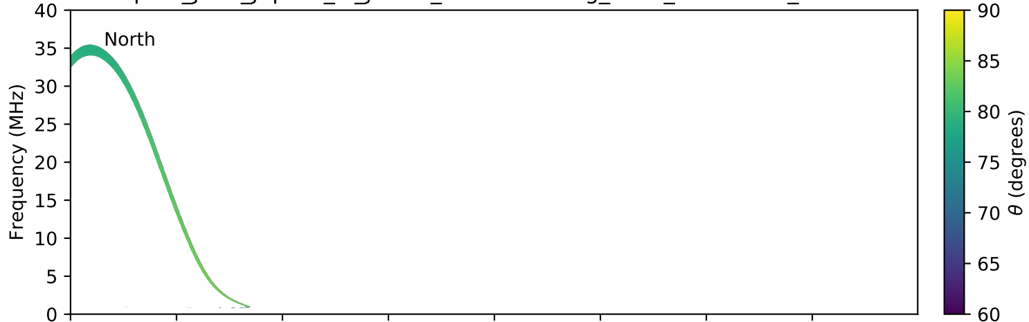
expres_juno_jupiter_io_jrm09_lossc-wid1deg_3kev_20210627_v11.cdf
