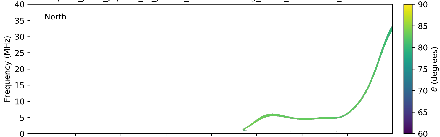
expres_juno_jupiter_io_jrm09_lossc-wid1deg_3kev_20210626_v11.cdf
