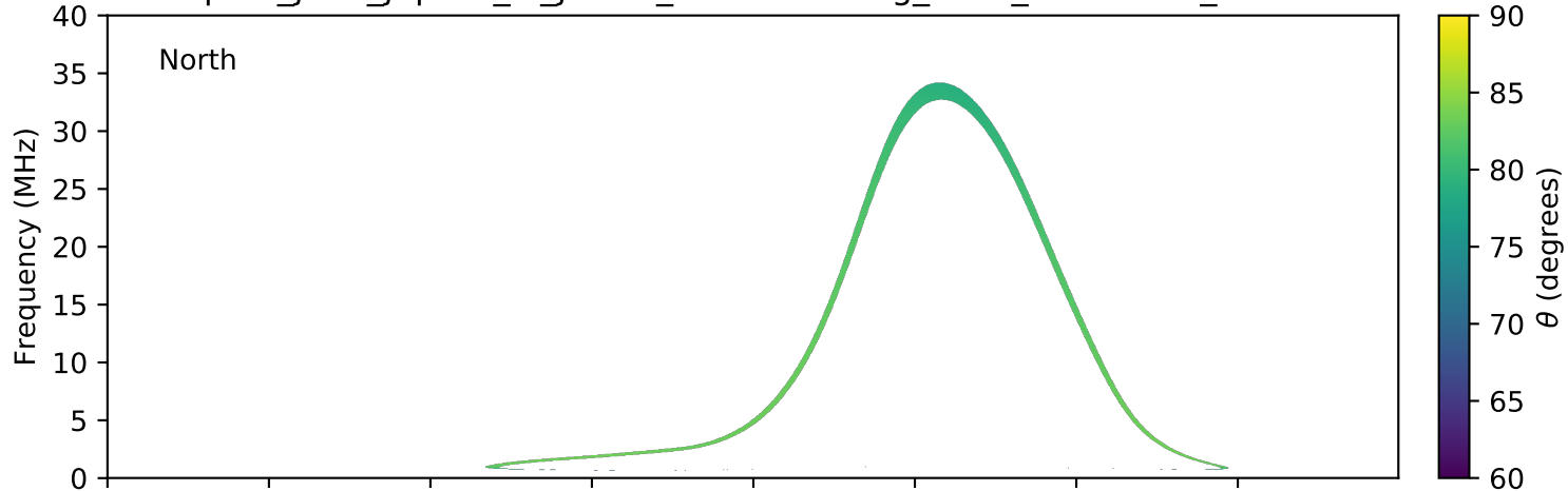
expres_juno_jupiter_io_jrm09_lossc-wid1deg_3kev_20210621_v11.cdf
