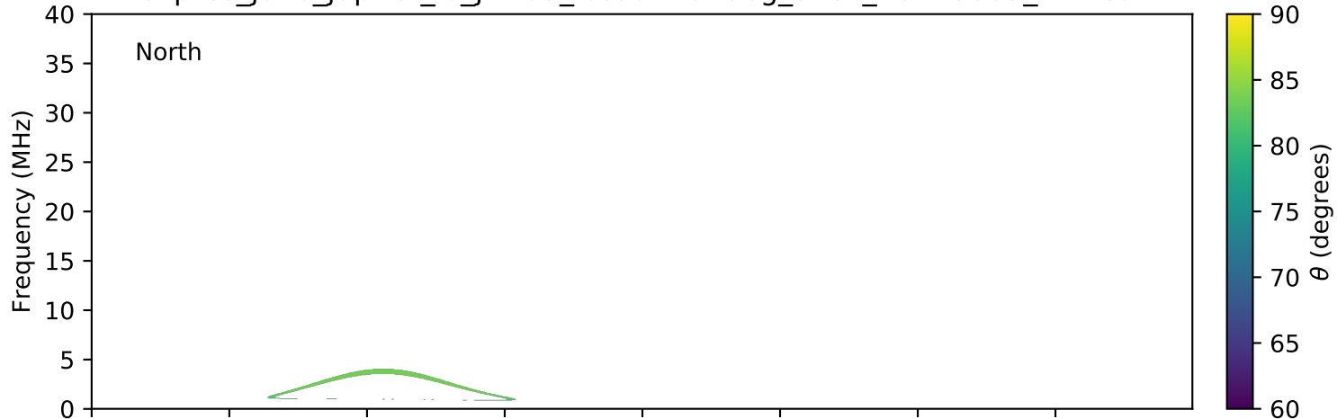
expres_juno_jupiter_io_jrm09_lossc-wid1deg_3kev_20210609_v11.cdf
