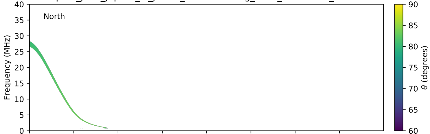
expres_juno_jupiter_io_jrm09_lossc-wid1deg_3kev_20210426_v11.cdf
