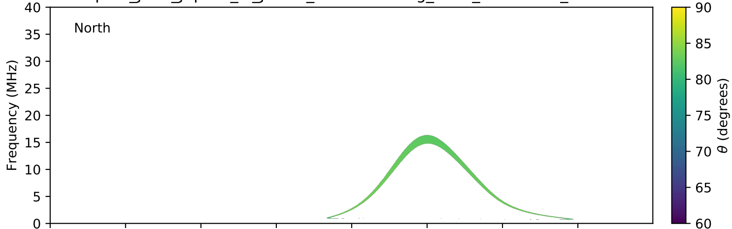
expres_juno_jupiter_io_jrm09_lossc-wid1deg_3kev_20210420_v11.cdf
