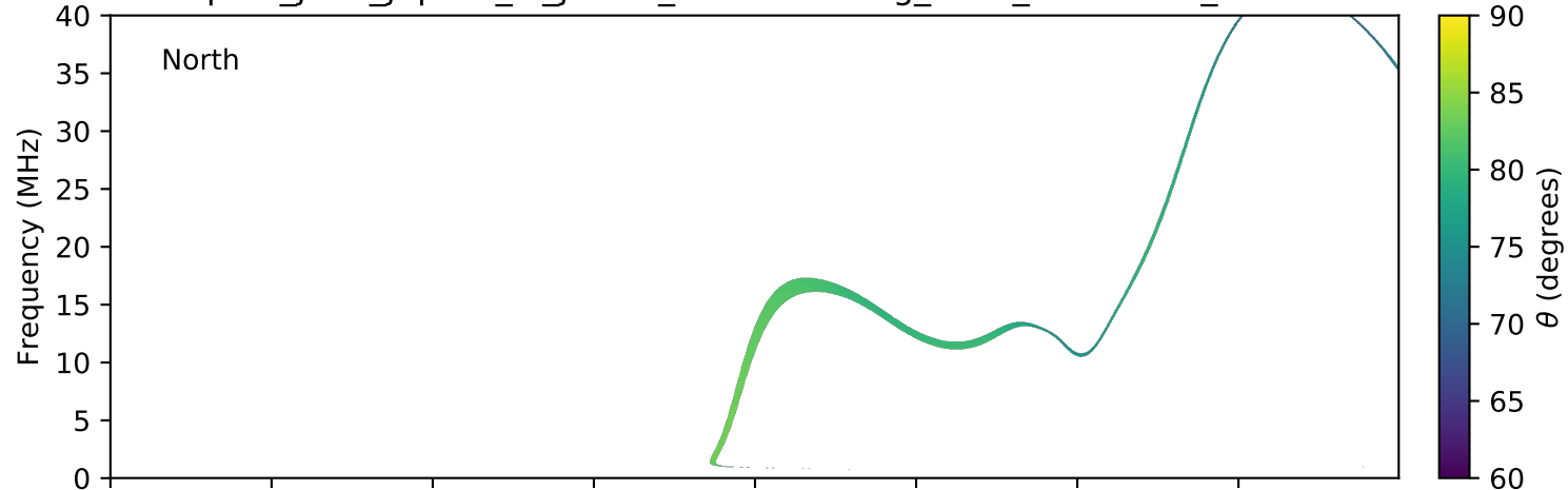
expres_juno_jupiter_io_jrm09_lossc-wid1deg_3kev_20210411_v11.cdf
