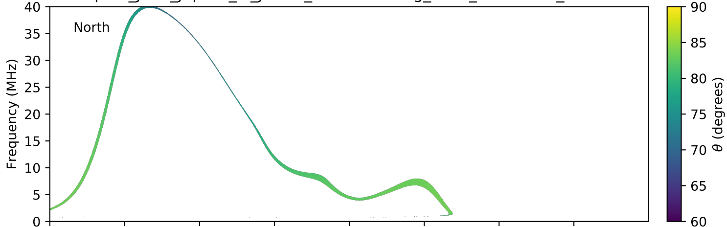
expres_juno_jupiter_io_jrm09_lossc-wid1deg_3kev_20210408_v11.cdf
