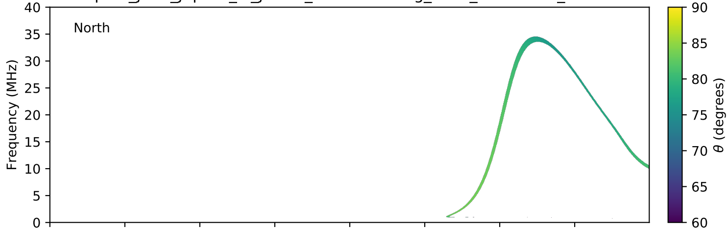
expres_juno_jupiter_io_jrm09_lossc-wid1deg_3kev_20210402_v11.cdf
