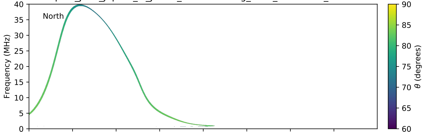
expres_juno_jupiter_io_jrm09_lossc-wid1deg_3kev_20210401_v11.cdf
