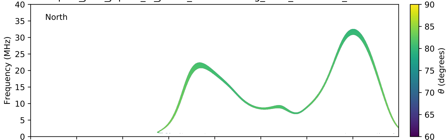
expres_juno_jupiter_io_jrm09_lossc-wid1deg_3kev_20210328_v11.cdf
