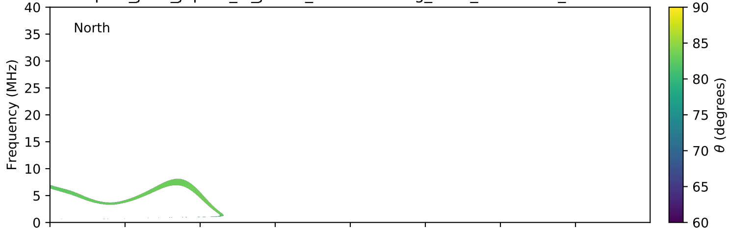
expres_juno_jupiter_io_jrm09_lossc-wid1deg_3kev_20210327_v11.cdf
