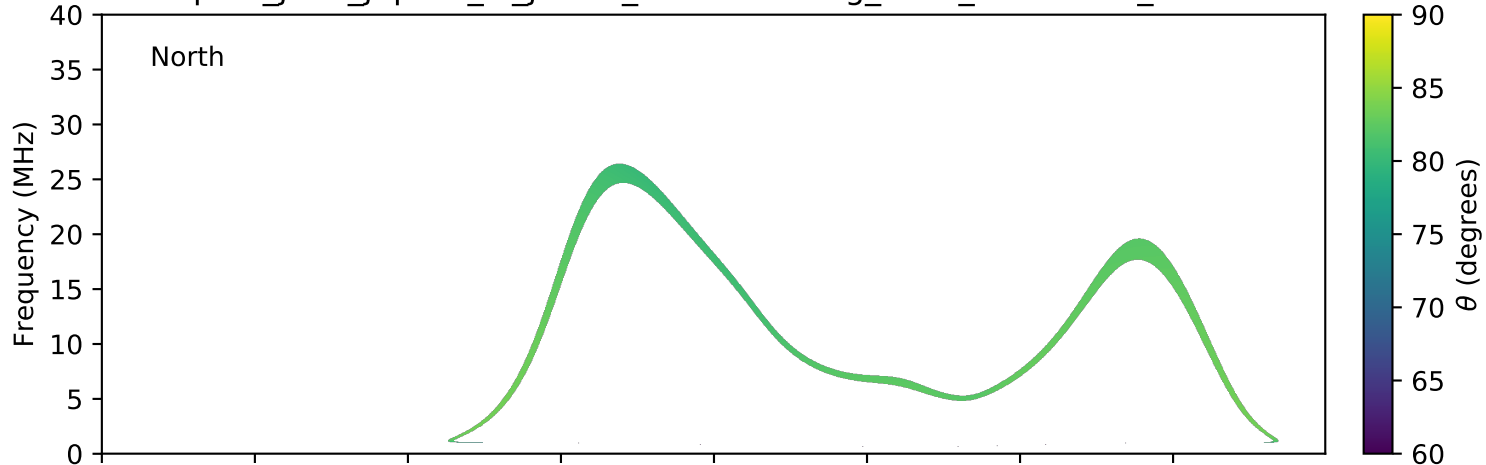
expres_juno_jupiter_io_jrm09_lossc-wid1deg_3kev_20210321_v11.cdf
